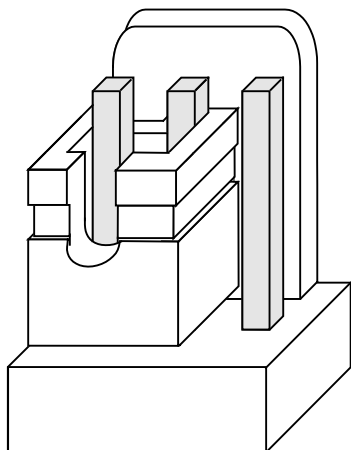
Rys. 20. Sposób założenia zworki na kołki portu RS-232 TTL.
